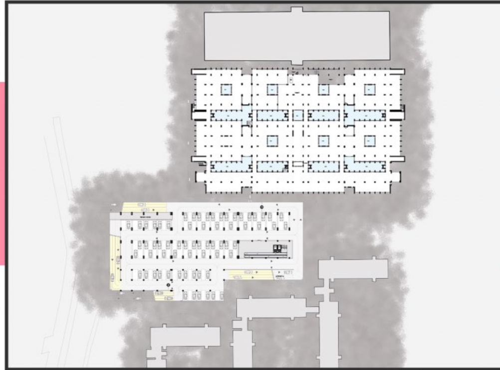
-3.00 KOT PLANI 125 ARAÇLIK OTOYAPAK
